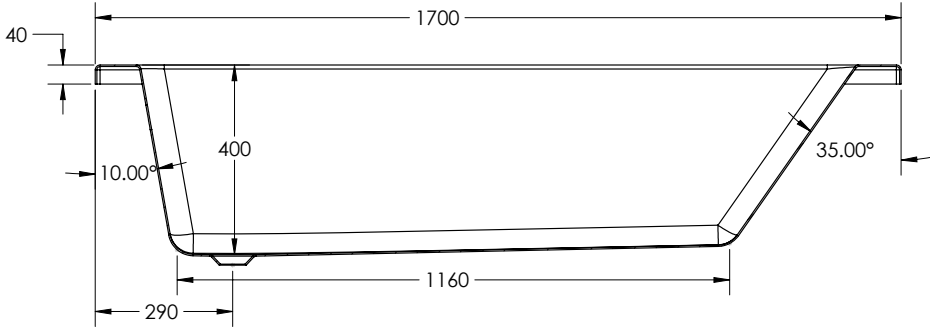
SECTION BA-BA SCALE 1 : 10
